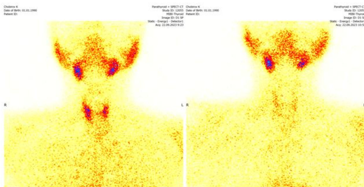
Рисунок 3.28. - Заключение сцинтиграфии
