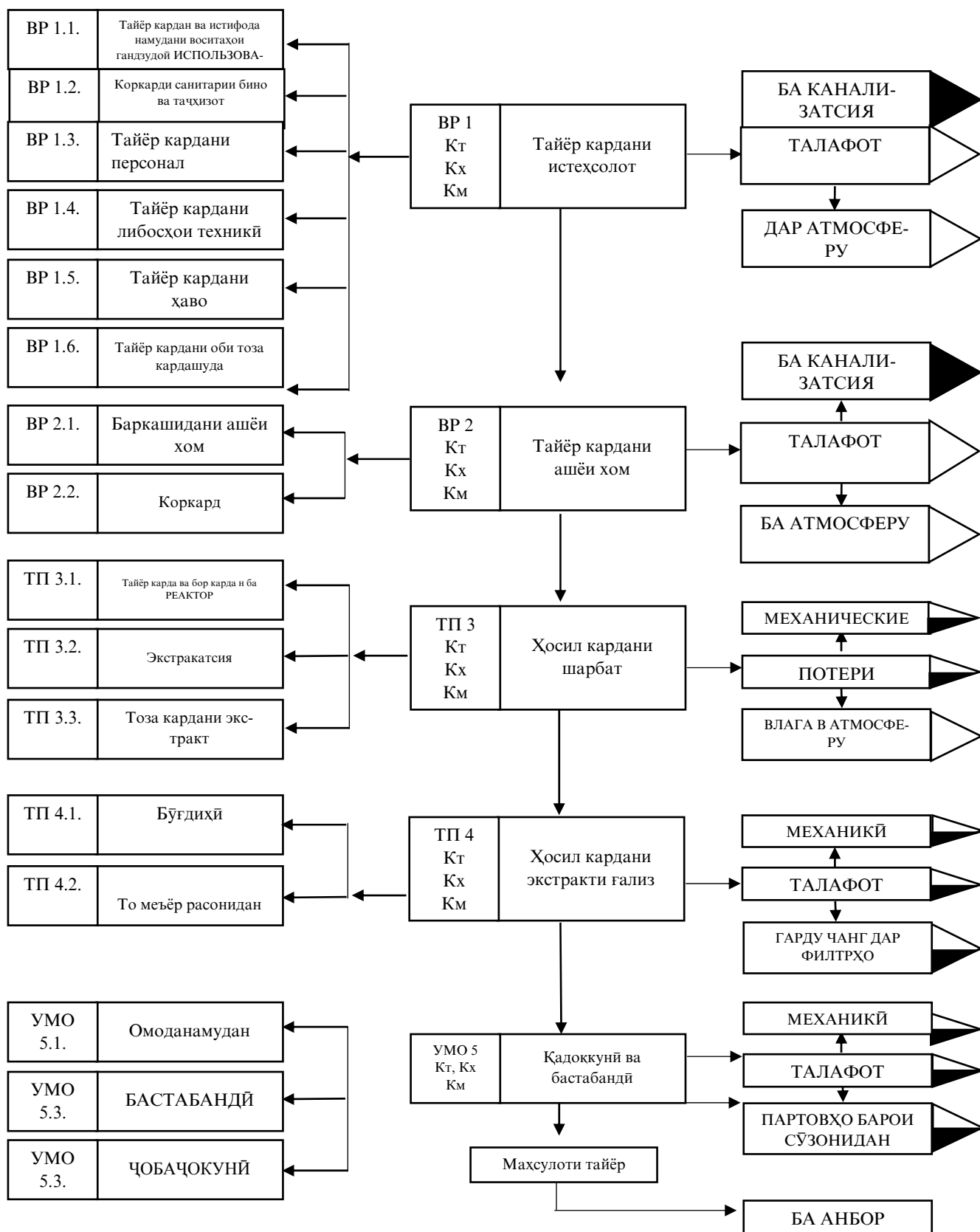
Расми 3- Нақшаи технологии истеҳсоли экстракти ғализ аз меваҳои хушки тути сафед (ТС-1) Кт, Кх, Км – муносибан назорати технологӣ, химиявӣ ва микробиологӣ
