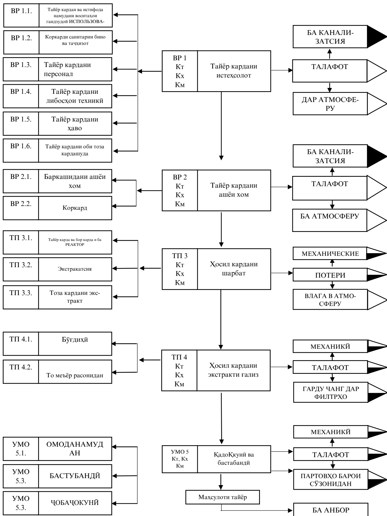
Расми 4- Нақшаи технологии истеҳсоли экстракти ғализ аз меваҳои хушкӣ тути сафед (ТС-2) К т , К х , К м – мутаносибан назарати технологӣ, химиявӣ ва микробиологӣ
