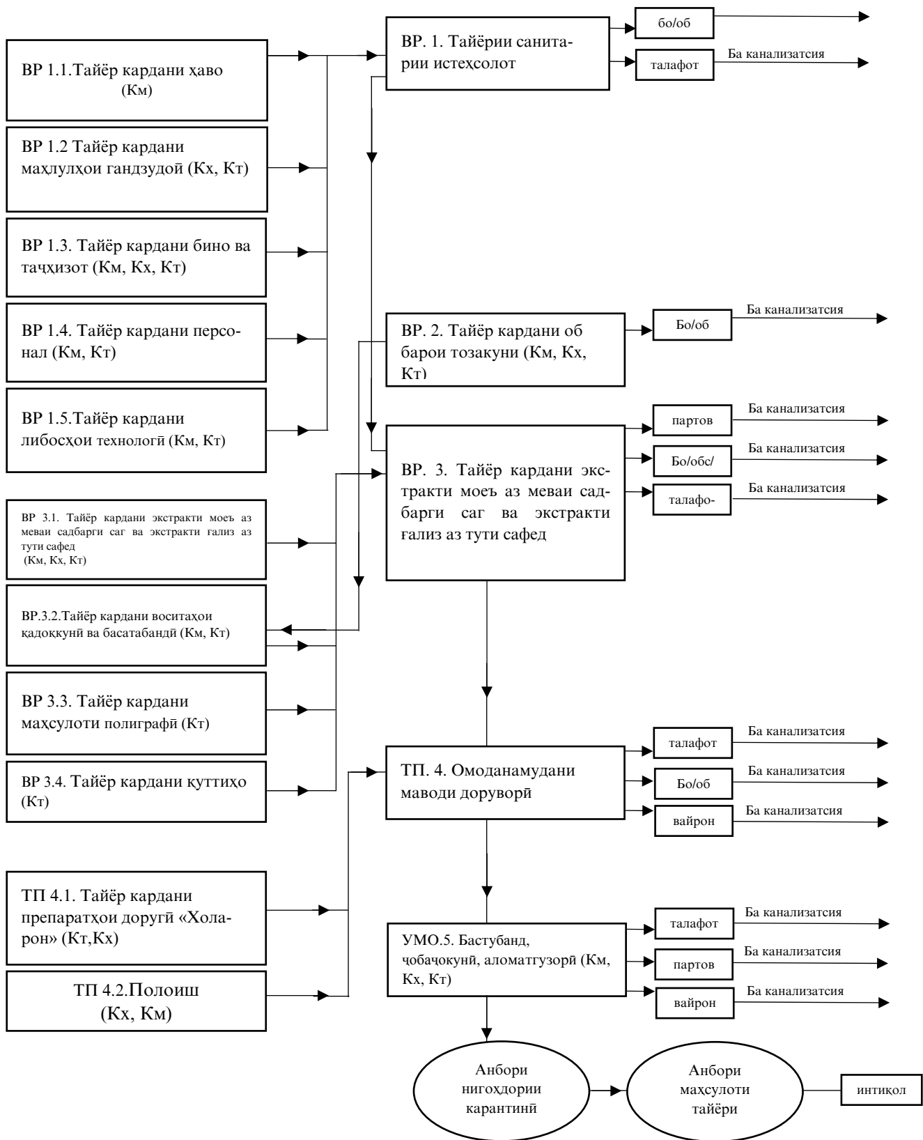
Расми 5-Нақшаҳои технологии истехсоли маҳлули ислоҳшудаи комплексӣ, ки экстракти меваи садбарги сағ ( лот. Rosa canina ) ва меваи тутӣ сафед дорад.
